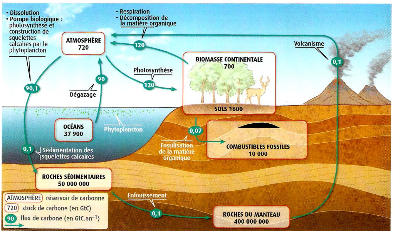
1 Le cycle naturel du carbone. GtC: milliard de tonnes de carbone.
