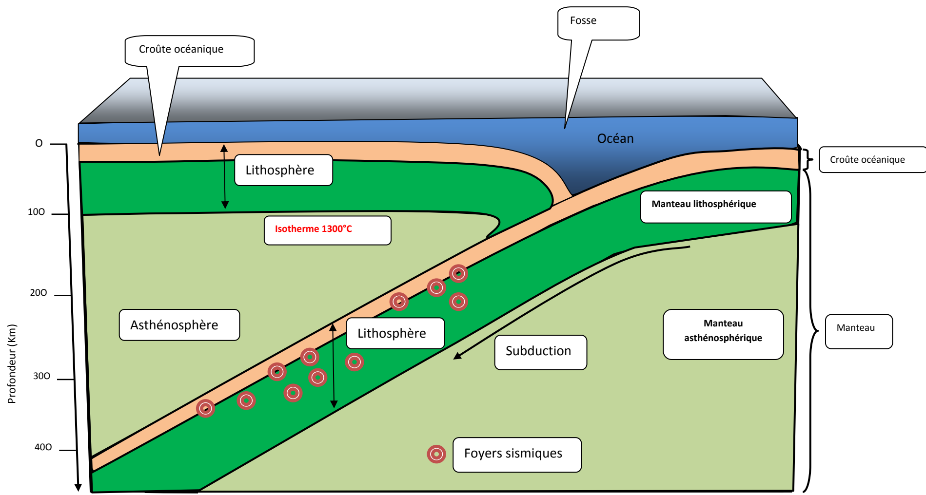
Le modèle de la subduction
