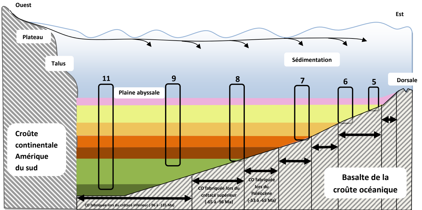
Coupe des fonds océaniques entre le Brésil et la dorsale de l'Atlantique sud. Répartition des sédiments océaniques
